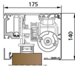
SL 45-S - Başkaları tarafından temin edilen kanat Kapı kanadı genişliği 50 - 90 mm
