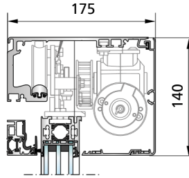
SL 45-S - Diğerleri tarafından temin edilen kanat ve bağlantı profili ile Kapı kanadı genişliği 50 - 90 mm
