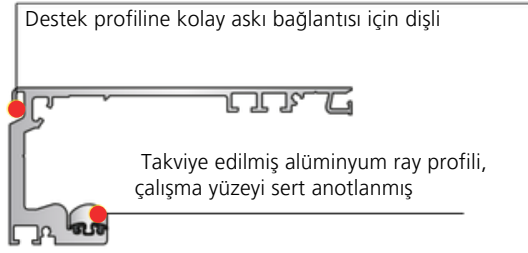
SL 45-S - standart (PSXP) Yan panel ve destek profili ile
