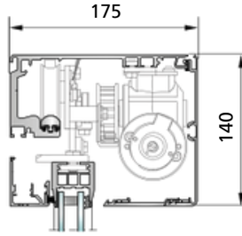
SL 45-S - standart (PSXP) Yan panel ve destek profili olmadan
