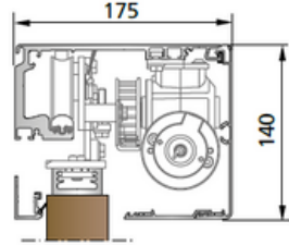
SL 45-S - Başkaları tarafından temin edilen kanat Kapı kanadı genişliği 50 mm'ye kadar
