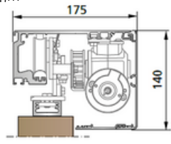
SL 45-S - Başkaları tarafından temin edilen kanat Kapı kanadı genişliği 50 - 90 mm
