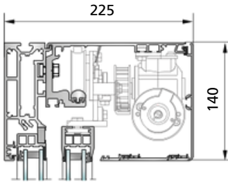
SL 45-S - standart (PSXP) Yan panel ve destek profili ile
