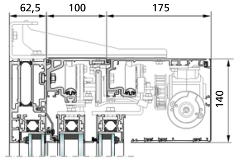
SL 45-T - ısı yalıtımlı (PST) Yan panel ve destek profili ile
