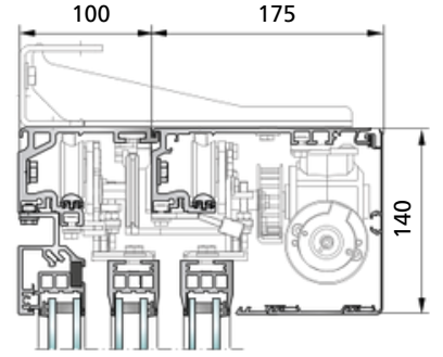
SL 45-T - ısı yalıtımlı (PST) Yan panel ve destek profili ile
