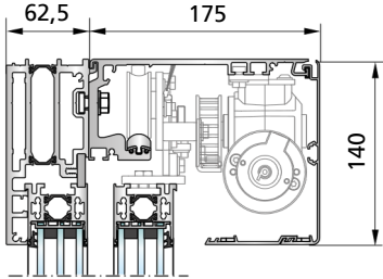
SL 45-S - Diğerleri tarafından temin edilen kanat ve bağlantı profili ile, kapı kanadı genişliği 50 mm'ye kadar
