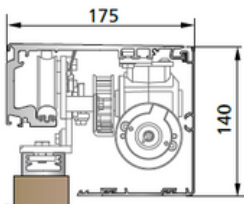
SL 45-S - Başkaları tarafından temin edilen kanat Kapı kanadı genişliği 50 mm'ye kadar
