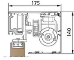
SL 45-S - Diğerleri tarafından temin edilen kanat Kapı kanadı genişliği 44 mm
