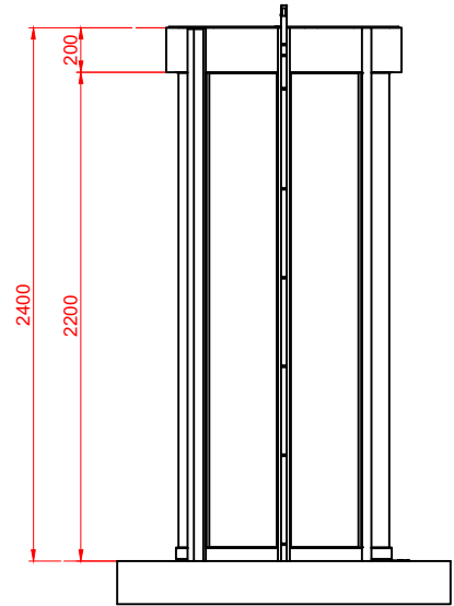
KESİT
